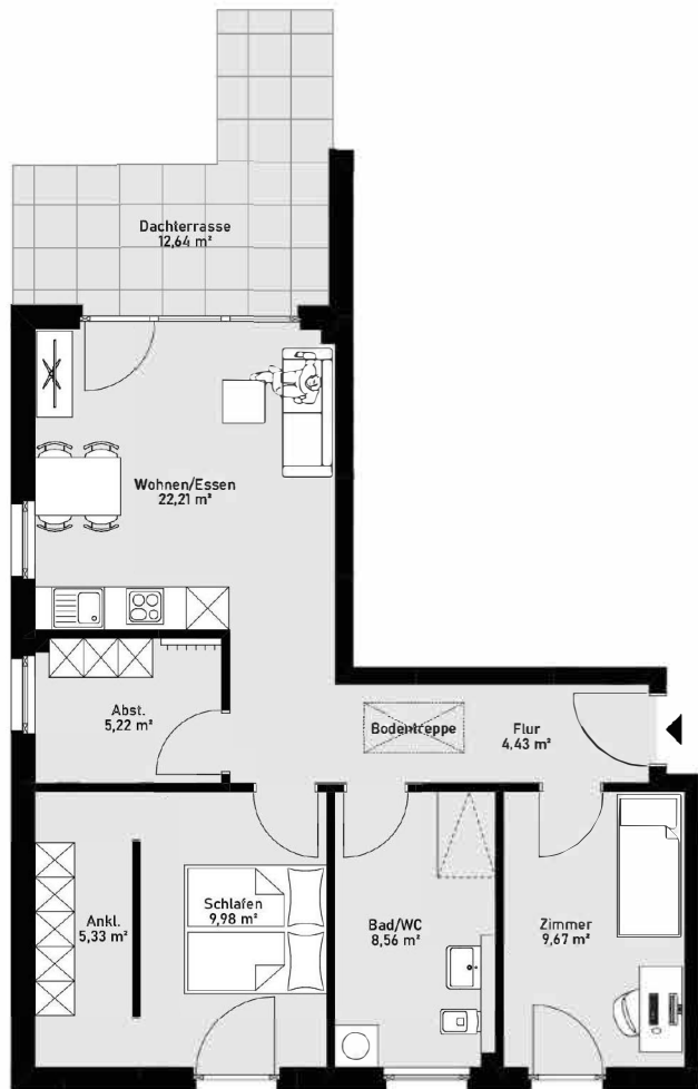
OBERGESCHOSS
